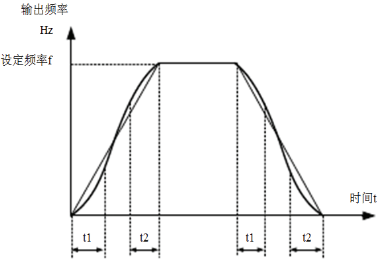
图 6-15 S 曲线加减速 A 示意图
