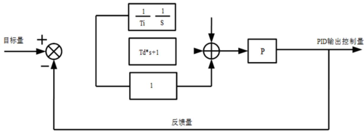
图 6-28 过程 PID 原理框图
