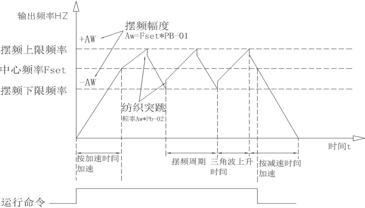
图 6-31 摆频工作示意图
