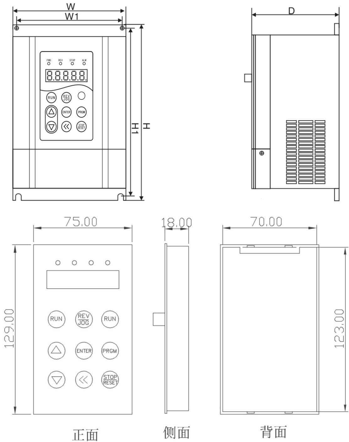
YP-B 面板尺寸图
