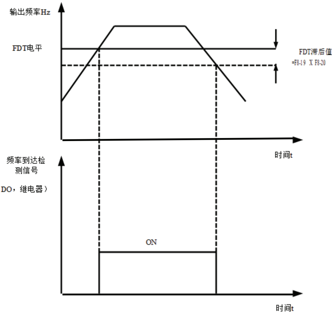
图 6-19 FDT 及频率达到功能示意图
