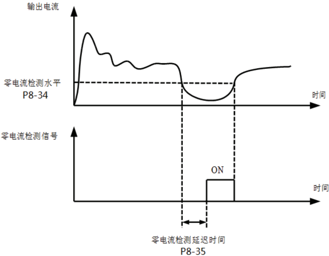
图 6-23 零电流检测示意图
