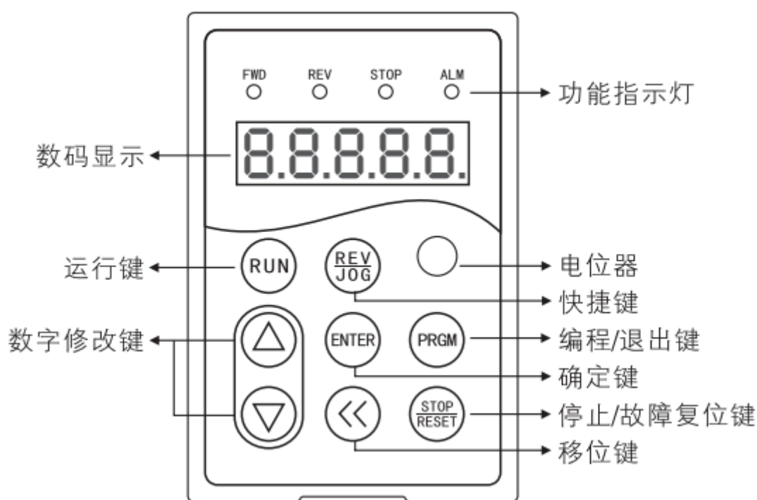
操作面板示意图
