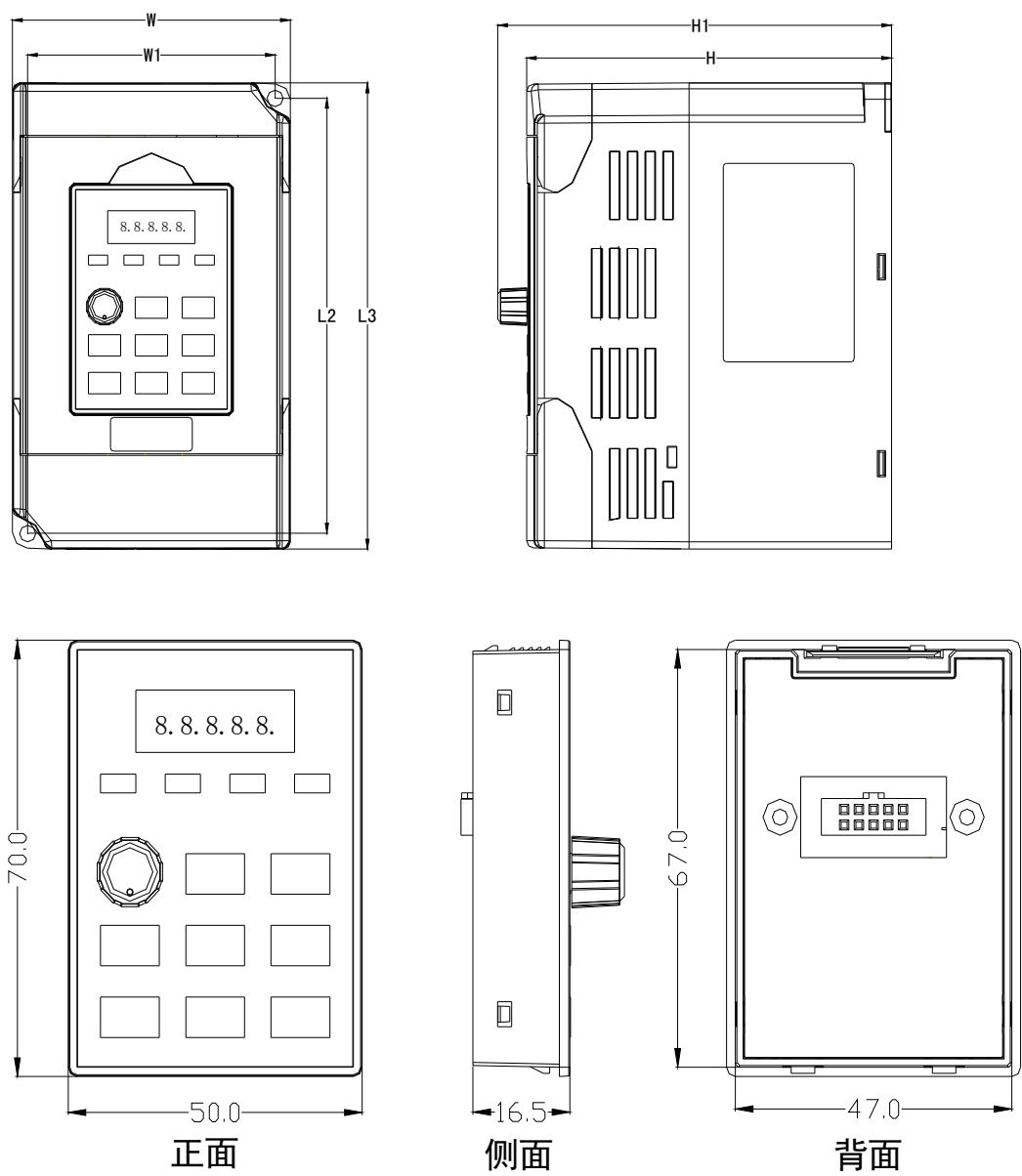
YP-A 面板尺寸图
