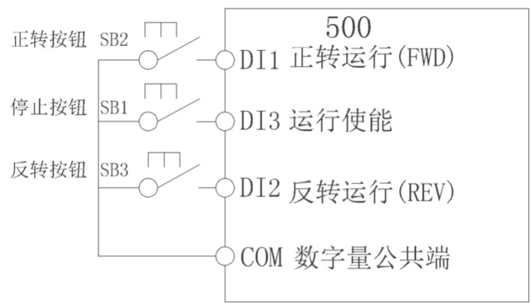
图 6-13 三线式控制模式 1
