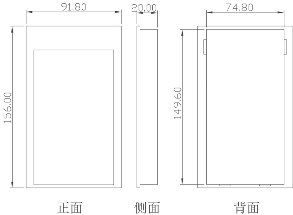
YP-B 托盘尺寸图
