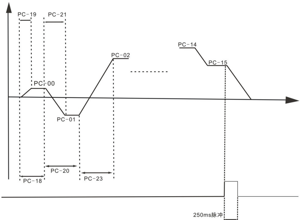
图 6-32 简易 PLC 示意图
