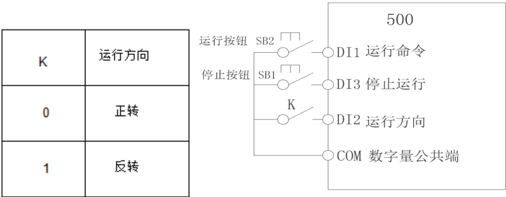
图 6-14 三线式控制模式 2
