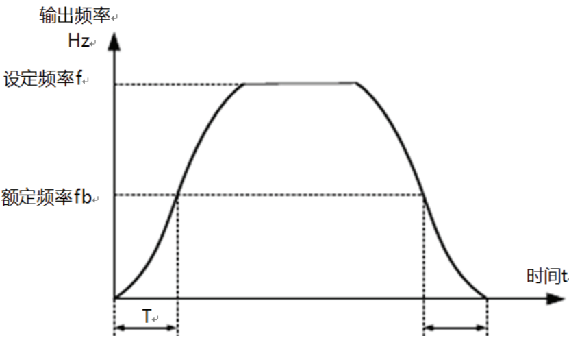
图 6-15 S 曲线加减速 B 示意图
